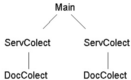
Figura 3.9. Hierarquia de fios de execução do Coleccionador . O Main lança um ServColect para a recolha de documentos de cada servidor. O ServColect lança um DocColect cada vez que recolhe um documento.
